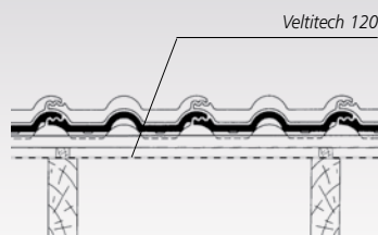
Dach nieocieplony
