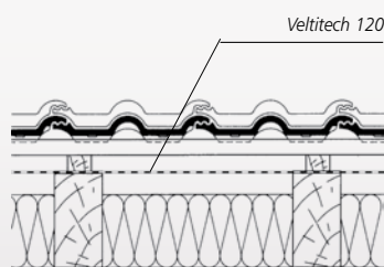
Dach ocieplony z zachowaną szczeliną wentylacyjną
